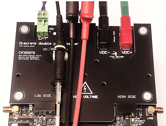
Figure 18. V_{GS} , V_{DS} , I_D Probes Connection
