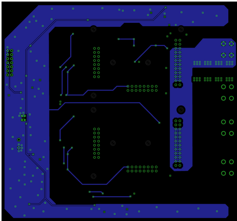
Figure 27. Bottom Layer
