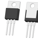
TO220-3 10.16x15.37x4.19, 2.54P CASE 221AL
