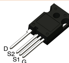
TO247-4L CASE 340CJ
