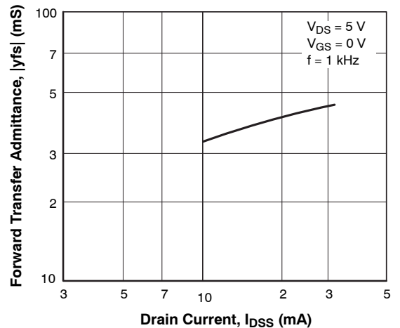
Figure 6. |y_{fs}| - I_{DSS}
