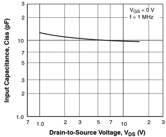
Figure 8. C_{iss} - V_{DS}
