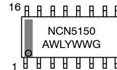
SOIC-16
