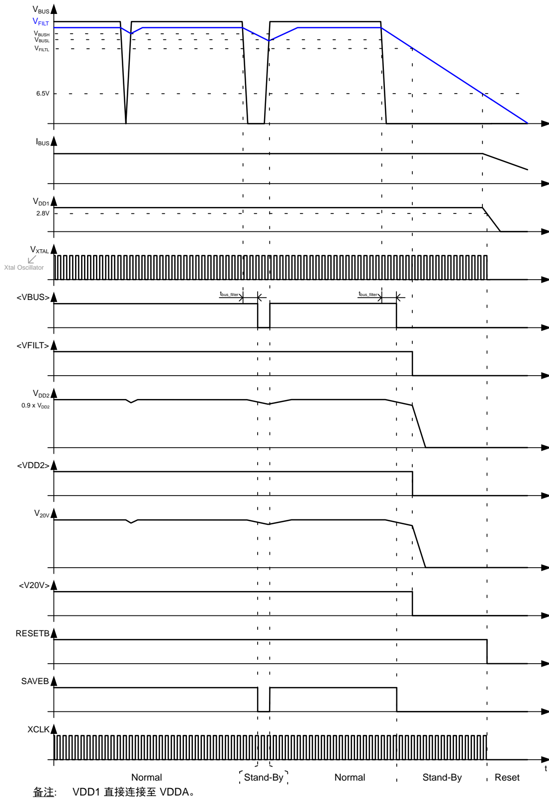
图 21. 关断行为
