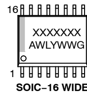
SOIC-16 WIDE
