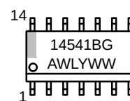
SOIC-14
