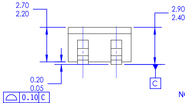
OPTION A - BEVEL EDGE
