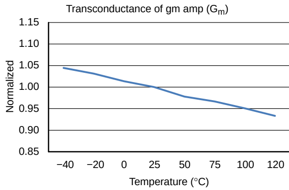
图 13. gm 放大器跨导与温度的关系
