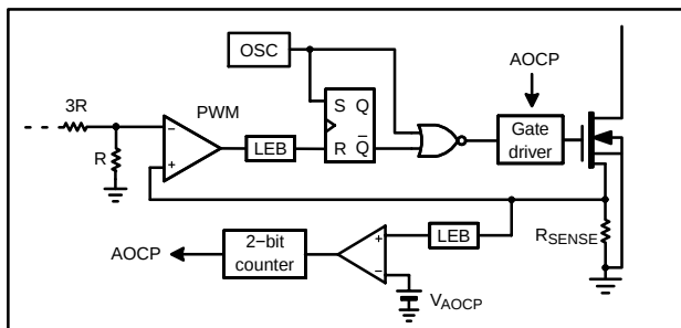
图 23. AOCP 电路
