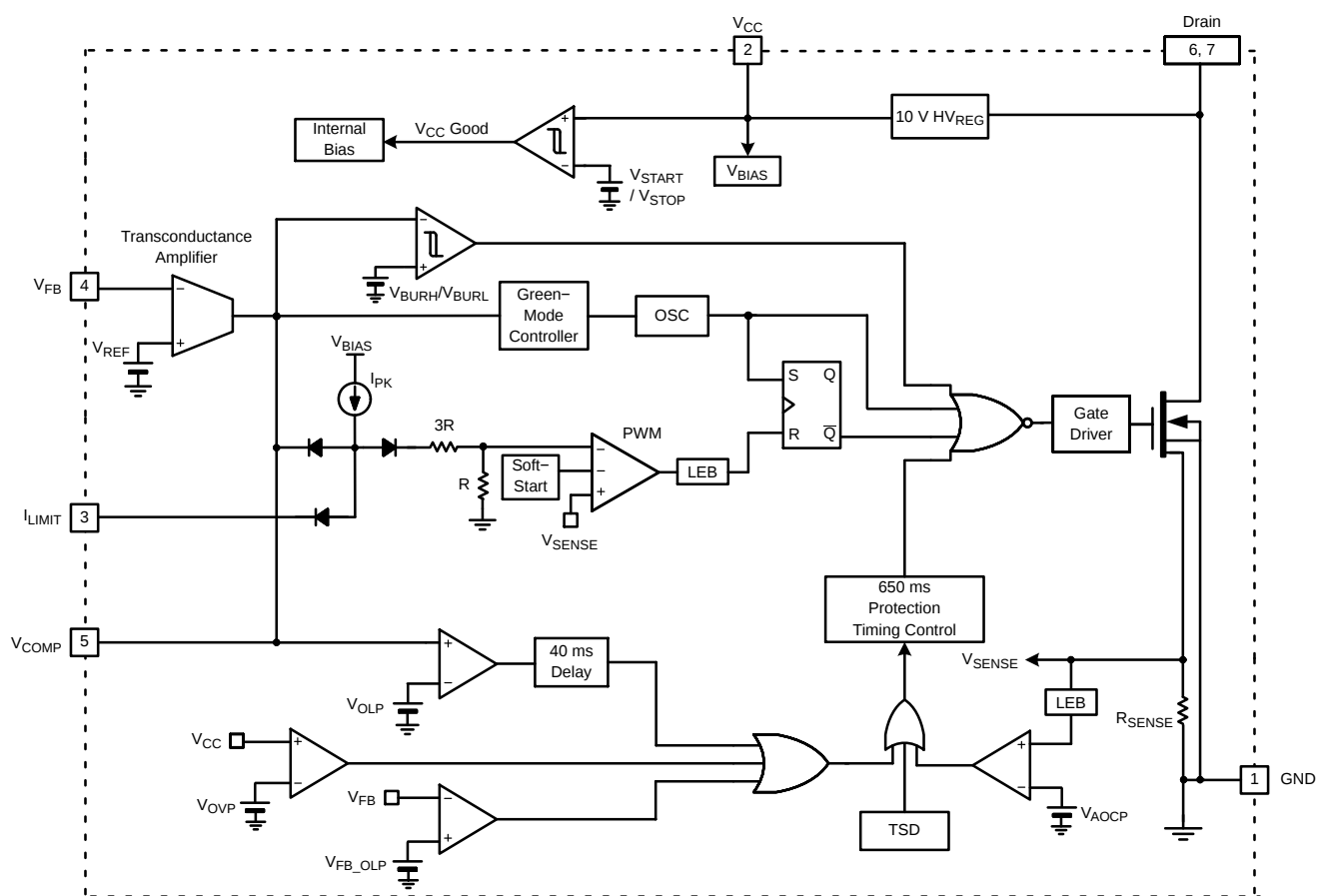
图 3. 内部框图
