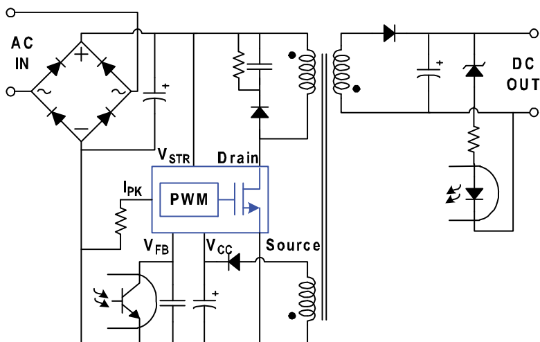
图 1. 典型应用图
