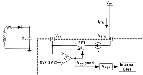
图 14. 启动电路
