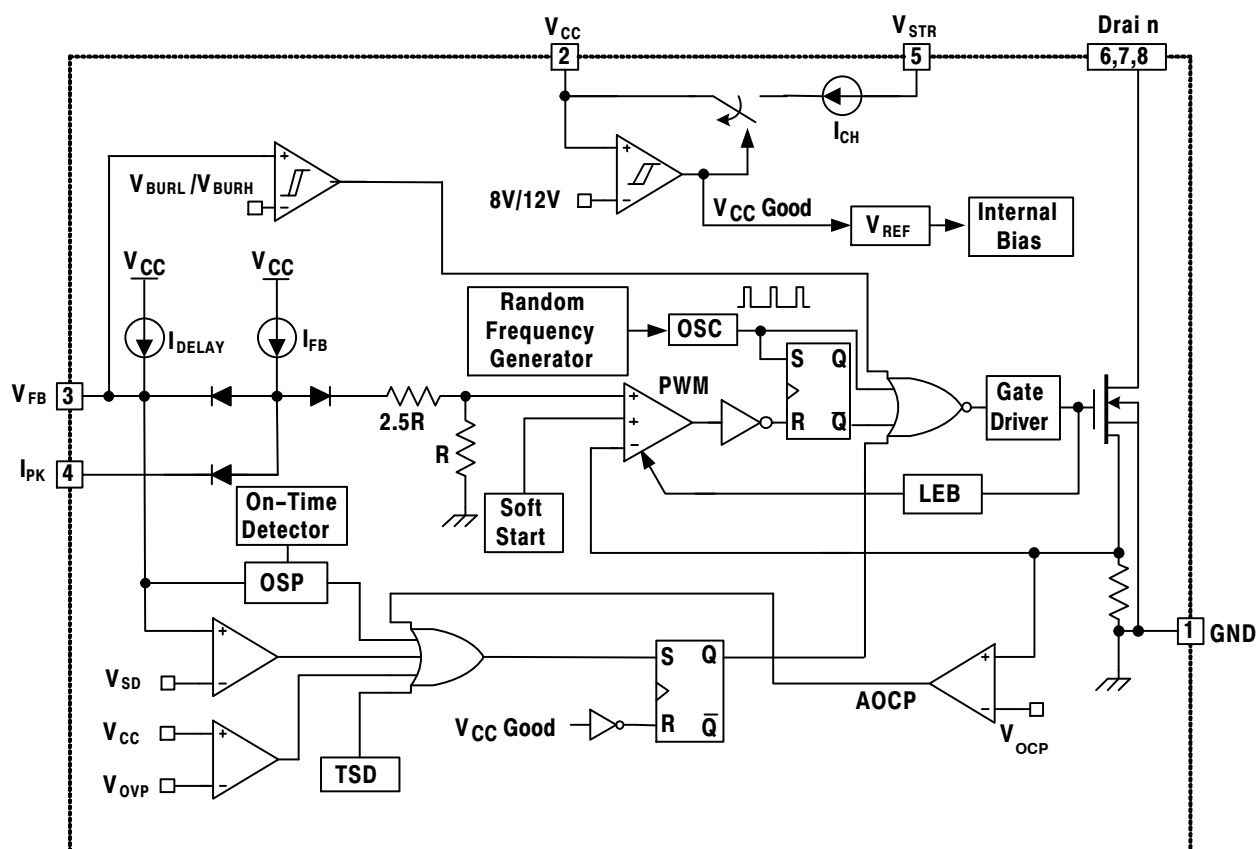
图 2. 内部框图
