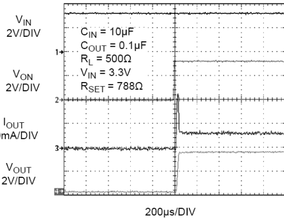
图18. t ON 响应
