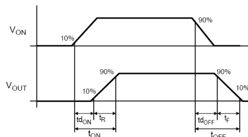
图27. 时序图
