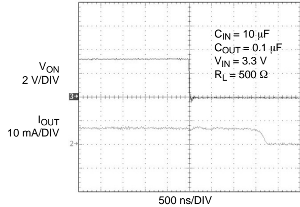
图 19. t_{dOFF} 响应
