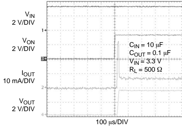
图 18. t_{dON} 响应
