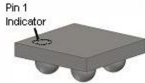
图 3. 1 x 1 毫米 WLCSP 封装, 凸块向下
