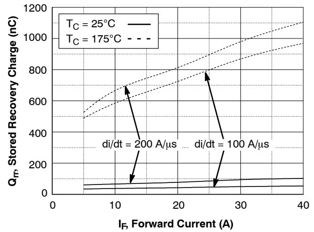
图 20. 存储电荷
