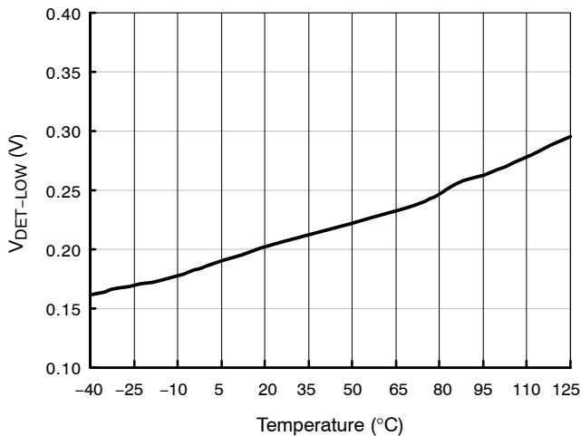
图 11. 箝位电压下限
