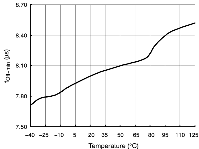
图 13. 最小关断时间 (V FB > V N )
