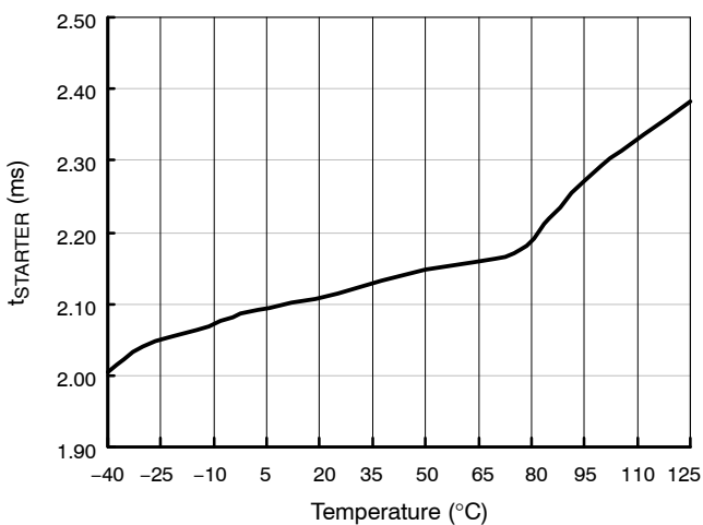
图 15. 启动计时器 (V FB < V G )
