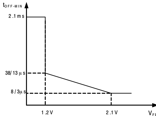
图 18. V_{FB} 与 t_{OFF-MIN} 曲线的关系
