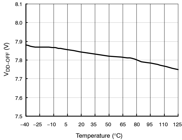
图 4. 导通阈值电压
