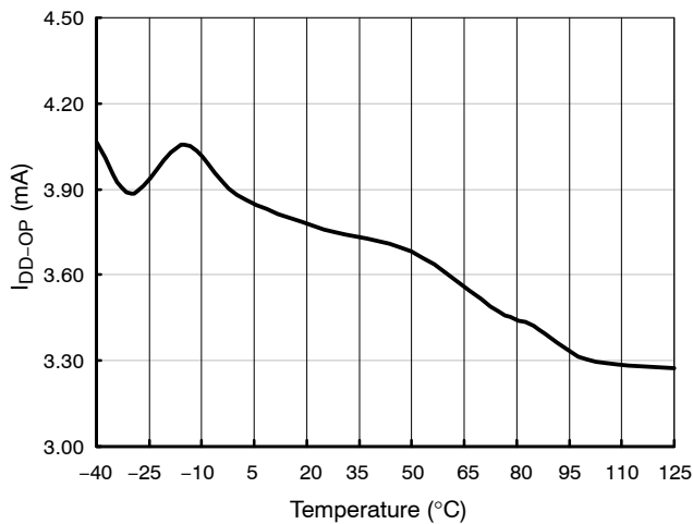
图 8. 工作电流
