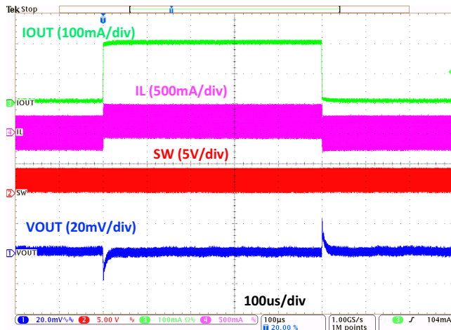
Figure 26. Load Transient 10\text{ mA} \leftrightarrow 200\text{ mA} , 1\text{ }\mu\text{s} Edge, FPWM Mode
