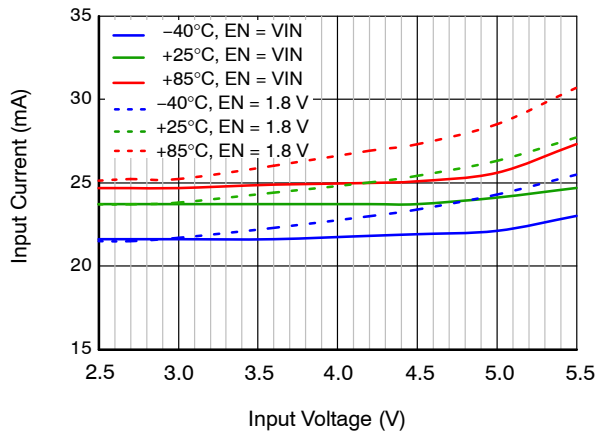
图 14. 静态电流与输入电压和温度的关系, 自动模式; EN = V_{IN} 实线, 点线表示 EN = 1.8\text{ V} ( -40^\circ\text{C} , +25^\circ\text{C} , +85^\circ\text{C} )
