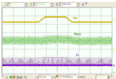
图 20. 线路瞬变, 3.3-3.9-3.3 V_{IN} , 10 \mu\text{s} 边沿, 36 mA 负载
