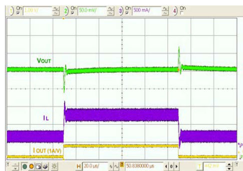
图 19. 负载瞬态, 200-800-200 mA, 100 ns 边沿
