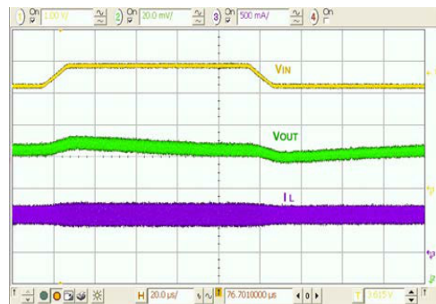
图 21. 线路瞬变, 3.3-3.9-3.3 V_{IN} , 10 \mu\text{s} 边沿, 600 mA 负载
