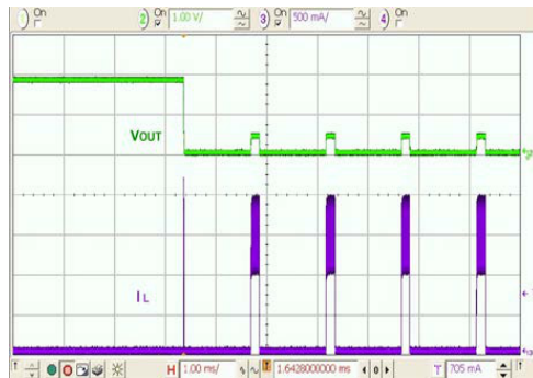
图 31. 250 mΩ 故障, 快速故障, 暂停, FAN53611
