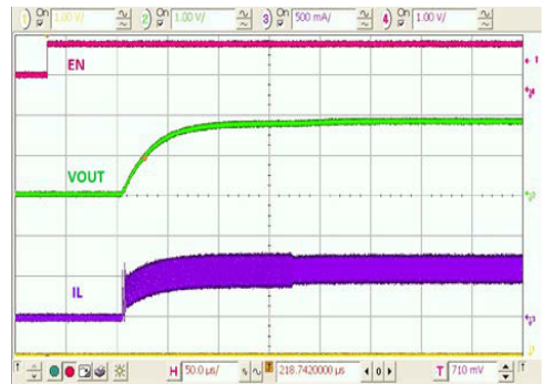
图 25. 启动, 3\text{ }\Omega 负载
