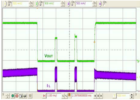
图 28. 过流, 负载增加过去电流限制, FAN53601
