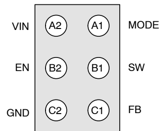
图 3. 焊球仰视图
