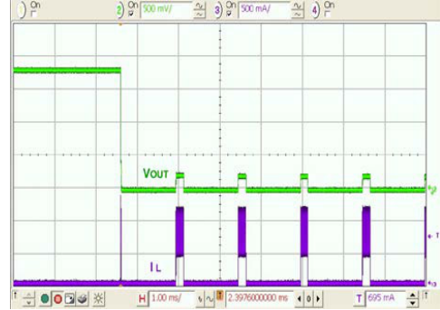
图 29. 250 mΩ 故障, 快速故障, 暂停, FAN53601
