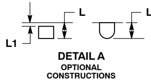
UDFN10 2.5x1, 0.5P CASE 517BB ISSUE O
