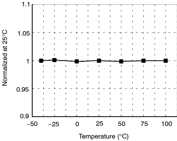
图 6. 高侧 V CC (HV CC ) 开始与温度的关系
