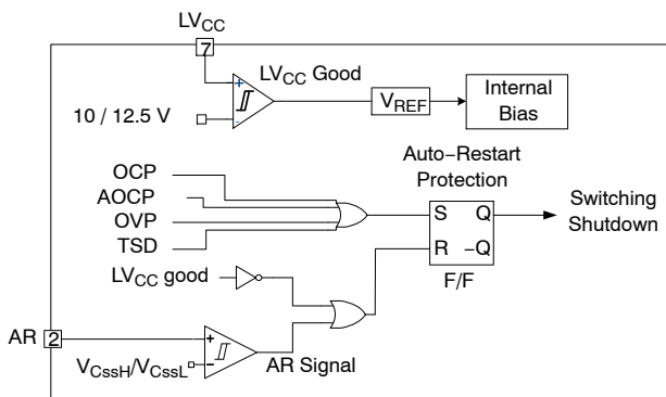
图 22. 保护框图
