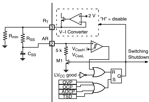
图 20. AR 引脚的内部框图
